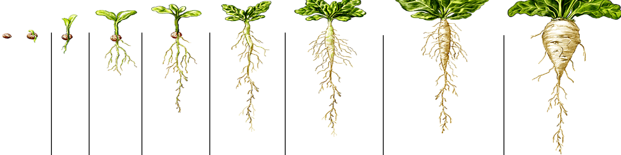
НАБУХАНИЕ ПРОРАСТАНИЕ ПОЯВЛЕНИЕ ВСХОДОВ 2 наст. листа 4 наст. листа 6 наст. листьев 8 наст. листьев ВЕГЕТАТИВНОЕ РАЗВИТИЕ СПЕЛОСТЬ И УРОЖАИ
